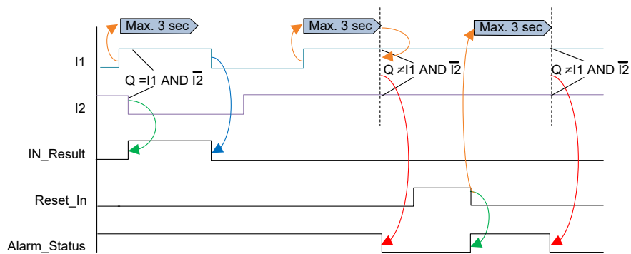
Fig. 43: Reset function 3
