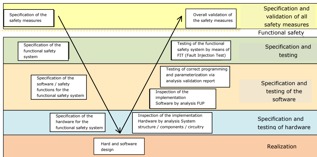
Fig. 64: V model
