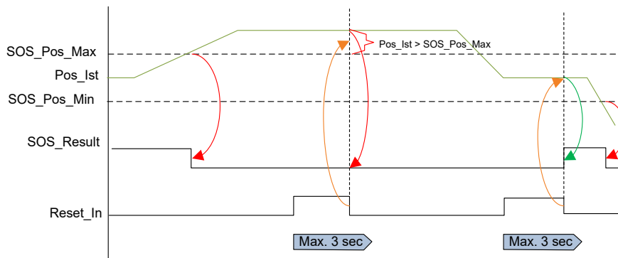
Fig. 41: Reset function 1
