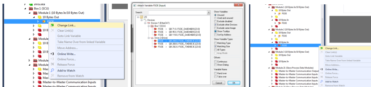
Fig. 51: TwinCAT - linking
