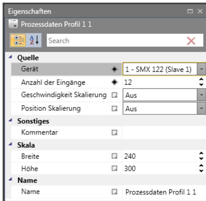
Abb. 39: Eigenschaftenfenster für Prozessdatenprofil 1
