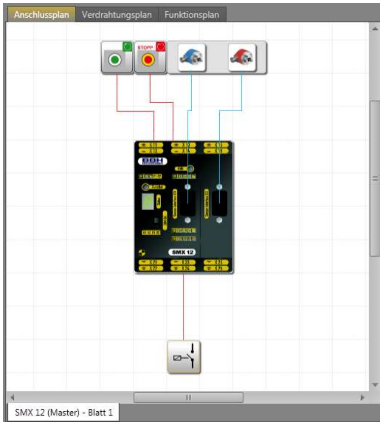
Abb. 16: Ansicht „Anschlussplan“
